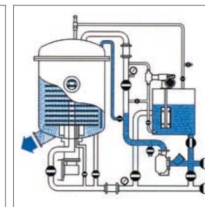
3. LAVAGGIO/ Washing
