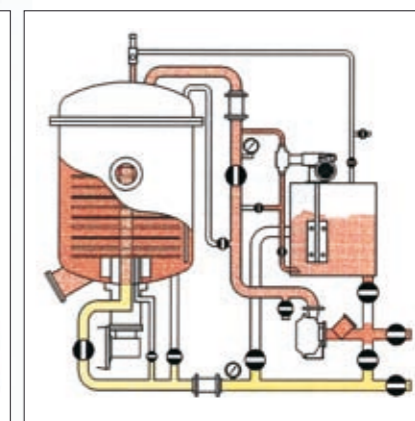
2. FILTRAZIONE/ Filter
